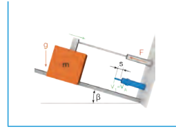
L9. Abwärts bewegte Masse mit entgegenwirkender Antriebskraft auf einer schiefer Ebene
