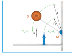
R3. Abwärts schwenkende Masse mit Antriebsmoment b) bei vertikaalem Aufprall
