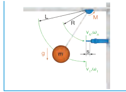
R3. Abwärts schwenkende Masse mit Antriebsmoment a) bei horizontalem Aufprall
