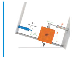
L11. Aufwärts bewegte Masse mit Antriebskraft auf einer schiefer Ebene
