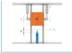
L4. Aufwärts bewegte Masse mit Antriebskraft
