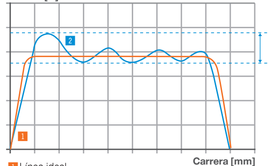
1 Línea ideal 2 PowerStop
