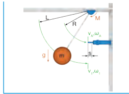
R2. Masa oscilante hacia abajo con par opuesto a) con impacto horizontal
