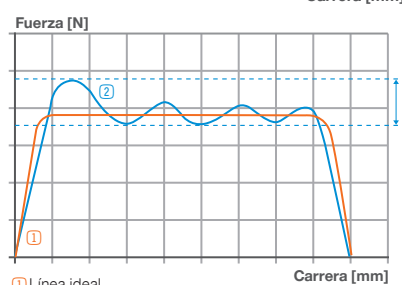
① Línea ideal ② PowerStop
