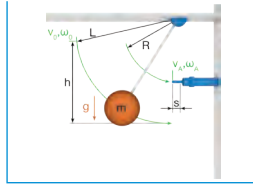
R1. Masa de oscilación libre a) con impacto horizontal
