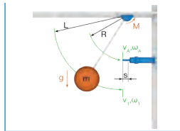
R3. Masa oscilante hacia abajo con par a) con impacto horizontal
