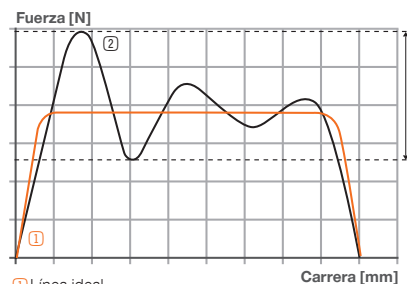
① Línea ideal ② Amortiguador convencional
