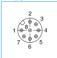
PIN - 할당
