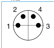
PIN分配
