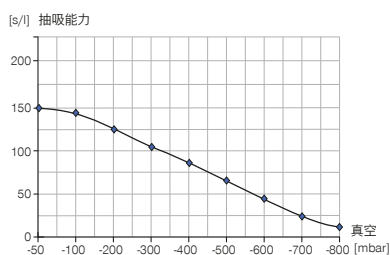
不同抽真空等级下的抽吸能力
