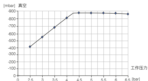
不同工作压力下可实现的真空度
