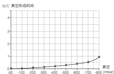
针对不同真空范围的真空形成时间
