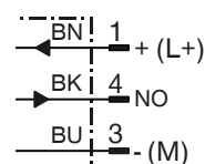
Schéma zapojenia
