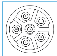
Occupazione PIN
