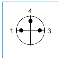
PIN - 할당
