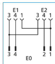
接线图
