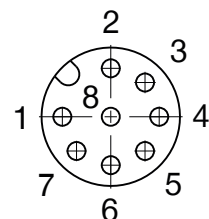
Obsadenie PIN-ov
