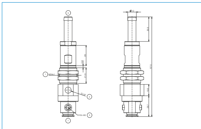
ZPS10/20/30-1B20-A/SS-H12
