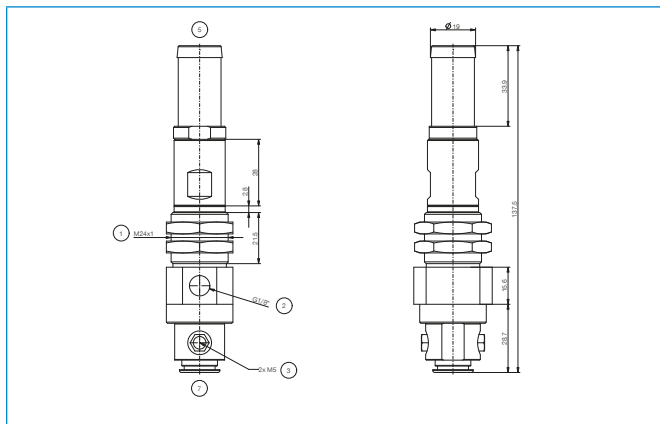
ZPS10/20/30-1B20-A/SS-H19
