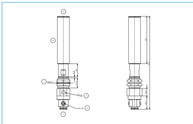
ZPS10/20/30-1B20-A/SS-S
