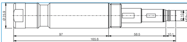
ZVCL303-NRV-HP2M25
