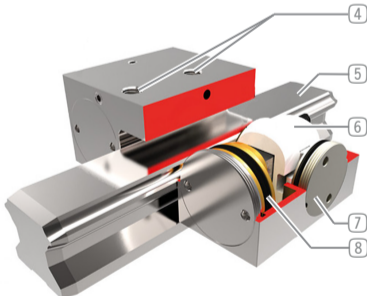
Abb. 2: Element der Serie MK im Schnitt
